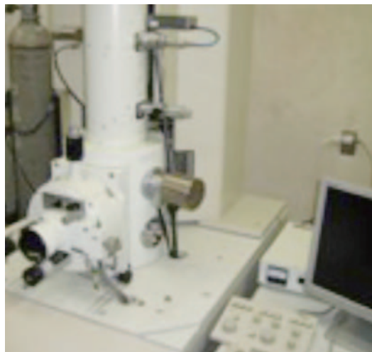
冷陰極フィールドエミッション電子銃と PC 制御による操作系を備えた走査電子顕微鏡
