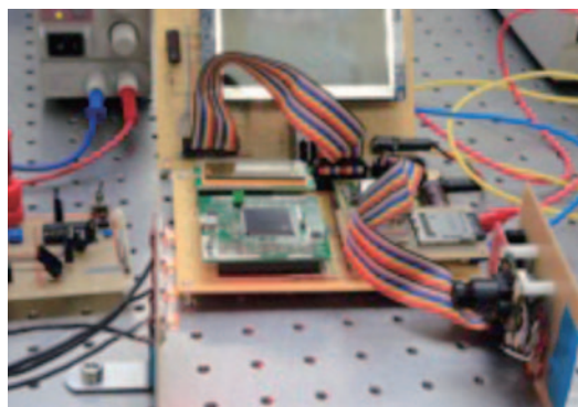
CMOSカメラと32bitマイコンを用いたLED可視光通信システム
